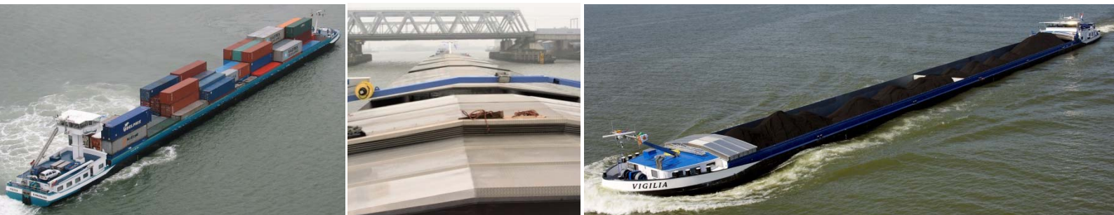
Container- och bulkpråmar kan flytta stora mängder gods från lastbilen och gatuutrymmet till pråmfartyg och inlandssjöfart. Fartygen är utrustade och specialbyggda för urbana miljöer med låga broar, trånga passager och enklare kajutrymmen. Foto: Johan Lantz och Vigilia Shipping BV
